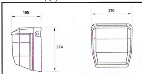
DIMENSION 尺寸
