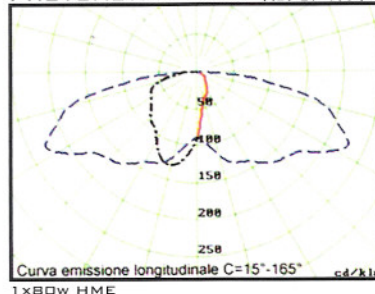
PHOTOMETRIC DATA 配光曲線圖
