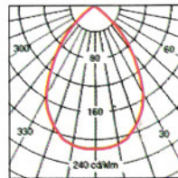
CAT.No. KI-480-226+CL CROSS LOUVER 2x26w PLC 十字交錯百葉
