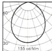
MII-6008 1x10W G24d-1
