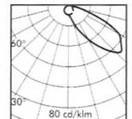
MII-6015 1x26W PLC
