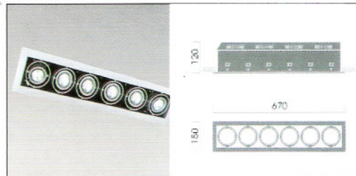
6-LAMPS 6 頭 MVI-1002-6
