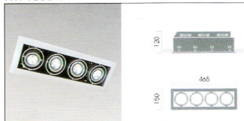
4-LAMPS SQUARE 方形 4 頭 MVI-1002-4S
