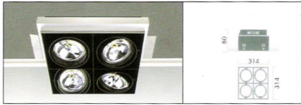
4-LAMPS SQUARE 方形 4 頭
