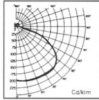
SINGLE LAMP W/ REFLECTOR 單管 + 反光片
