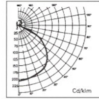
DOUBLE LAMP W/ REFLECTOR 孖管 + 反光片
