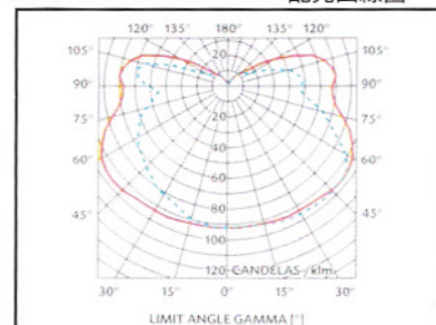
PHOTOMETRIC DATA 配光曲線圖
