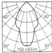
CAT.No. RI-1016-126 VERTICAL OPEN 1x26w PLC
